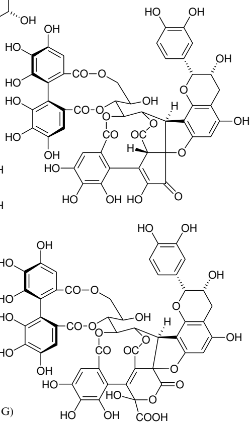
(217) (Camelliattannin F)
