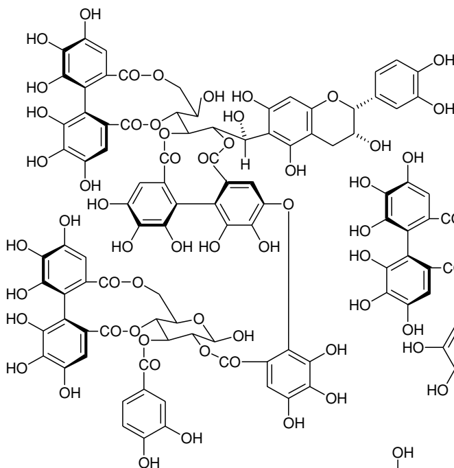
(216) (Camelliattannin D)
