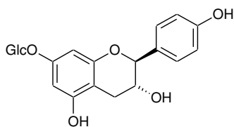
(73)
