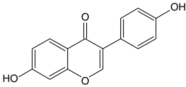
Genistein
