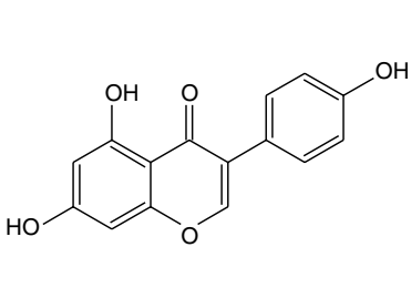
Genistein
