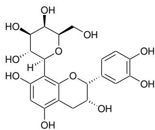
(77)
