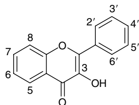
13.10
