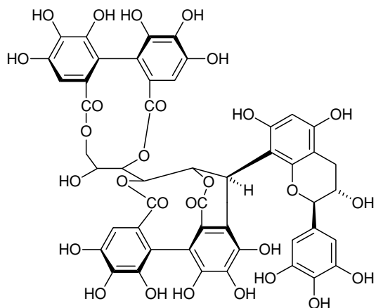
(213) Strobilanin
