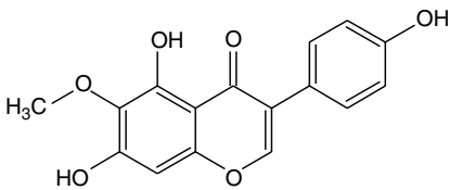
Glycitein
